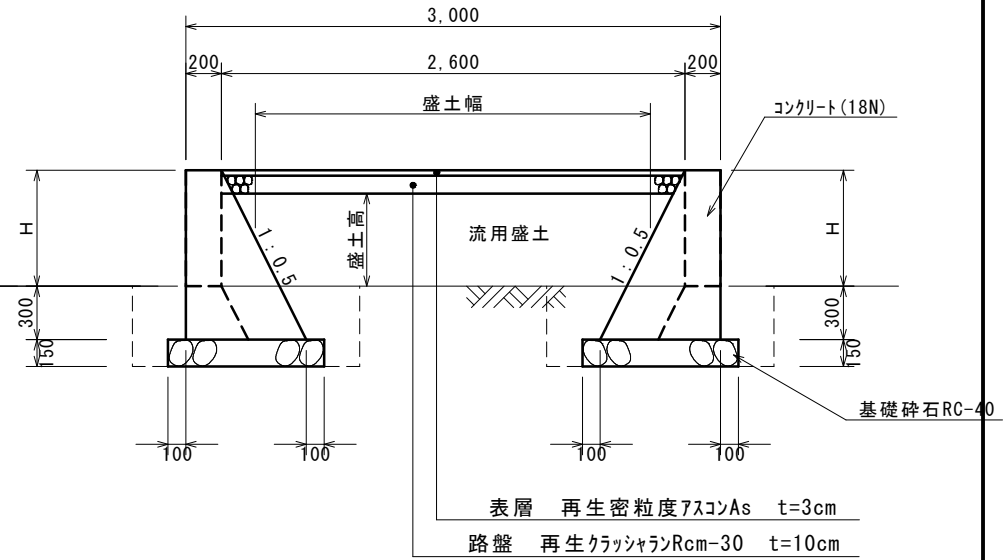
断面図
