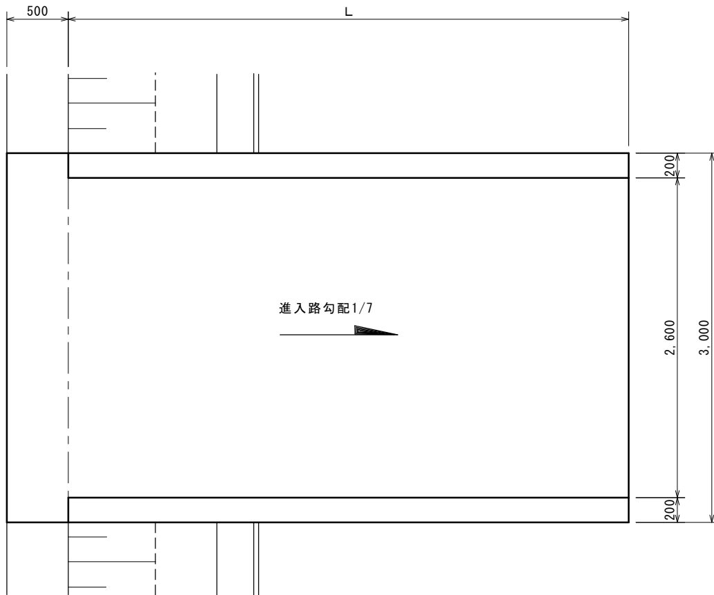
平面図
