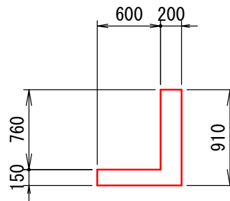
E-E断面 L=0.15m
