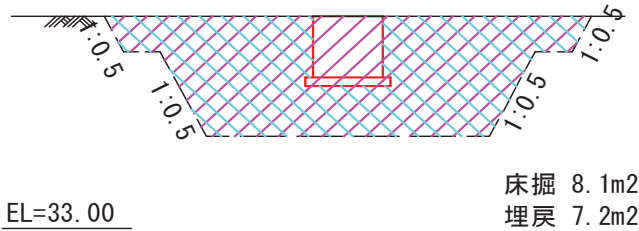
1-1 断面図
