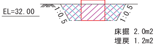
4-4 断面図
