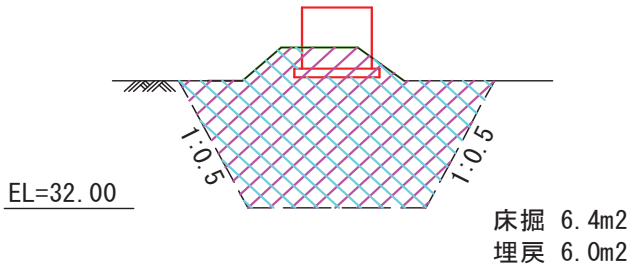
2-2 断面図
