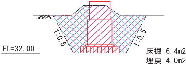
2-2 断面図
