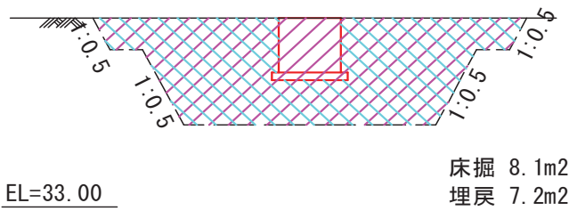
1-1 断面図
