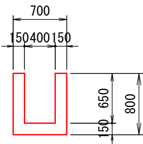
D-D断面 L=0.9m
