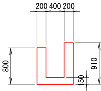
D-D断面 L=0.9m
