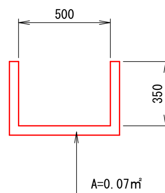
コンクリート取壊し鉄筋② B-B断面 L=0.15m
