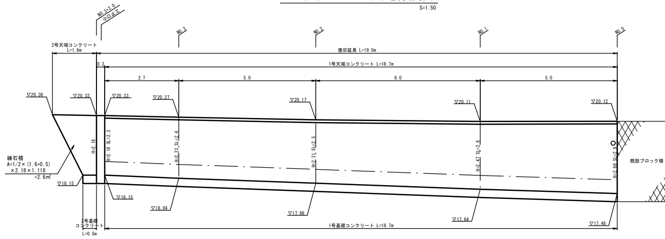
コンクリートブロック積展開図
