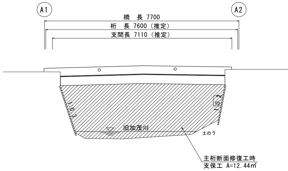
側 面 図
