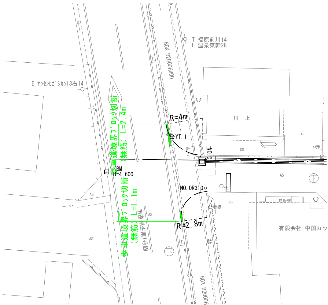
撤去工平面図
