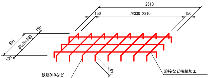
ジオセル展開補助枠(参考)
