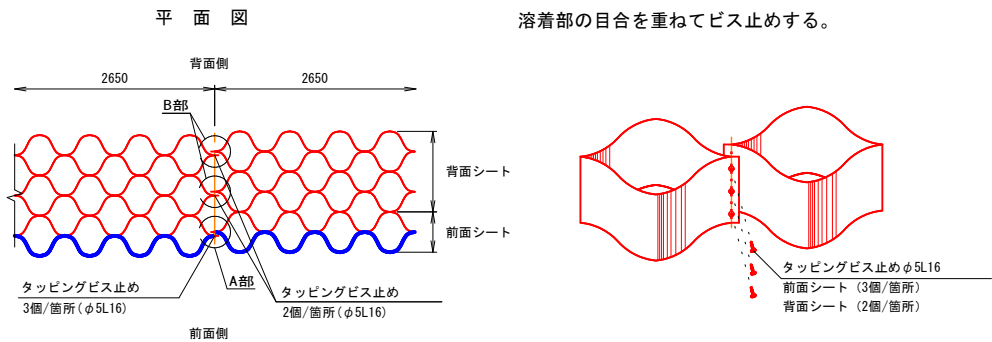
ジオセル相互接合部詳細
