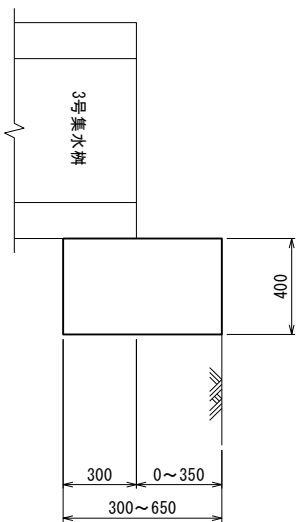
断面図
