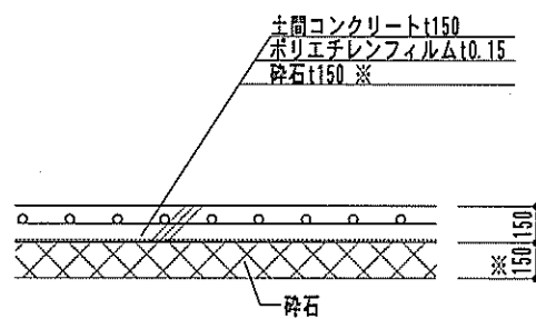
改修後 土間断面図 (家庭科室以外)
