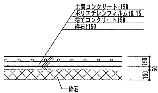
改修後 土間断面図 (家庭科室)
