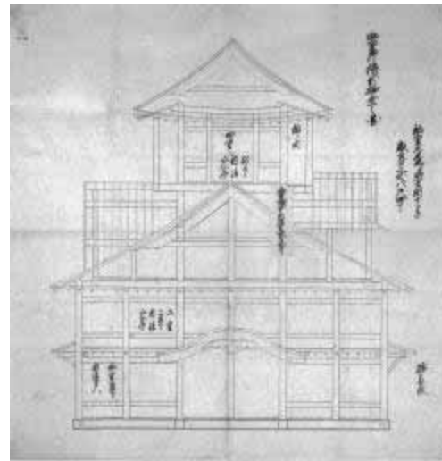
四重櫓絵図面入 2. 四重櫓
