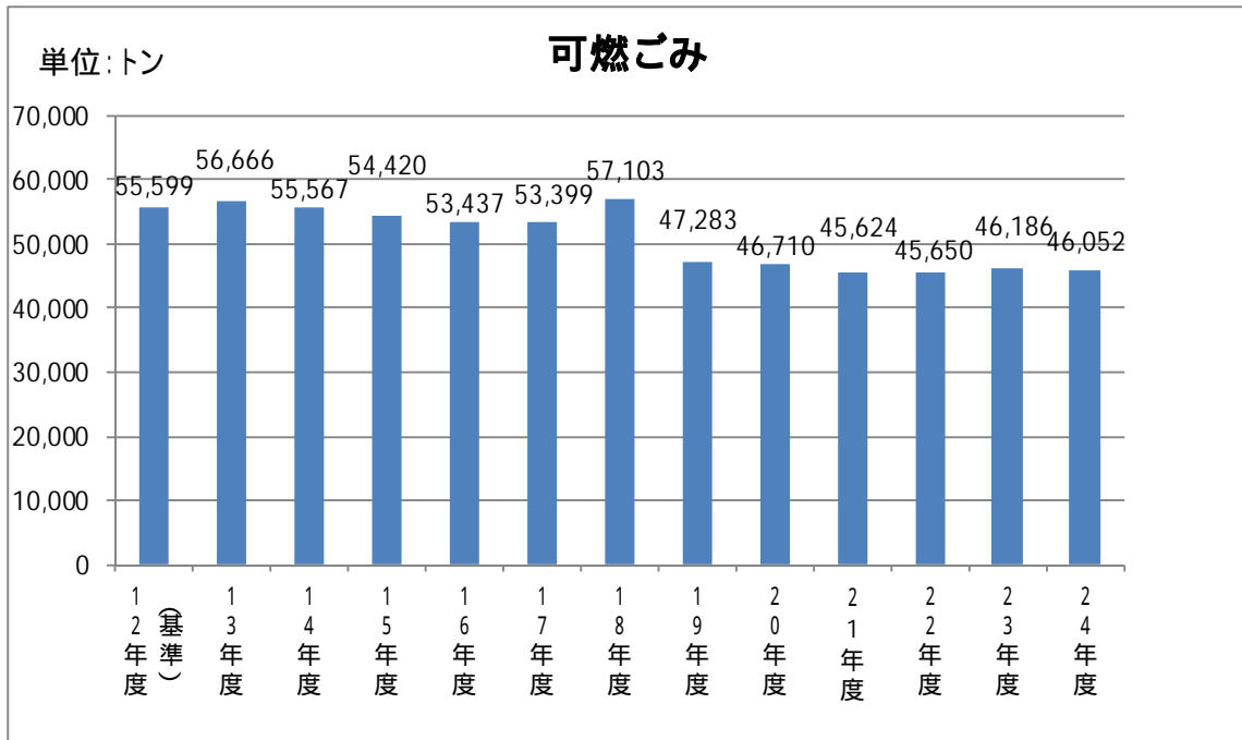
図-20 可燃ごみ処理量比較(平成12年度～24年度)
