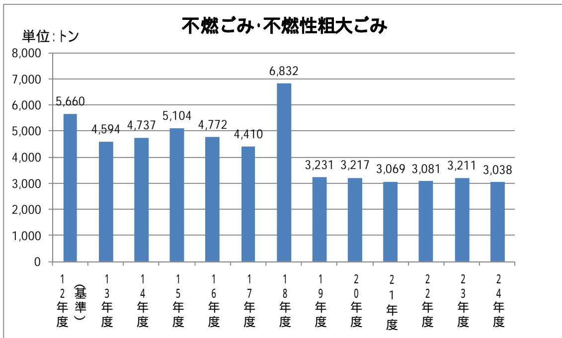
図-21 不燃ごみ・不燃性粗大ごみ処理量比較(平成12年度～24年度)
