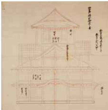
米子城四重櫓二十分一図（弘化4年）
