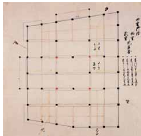
米子城四重櫓初重二重地差図（弘化4年）
