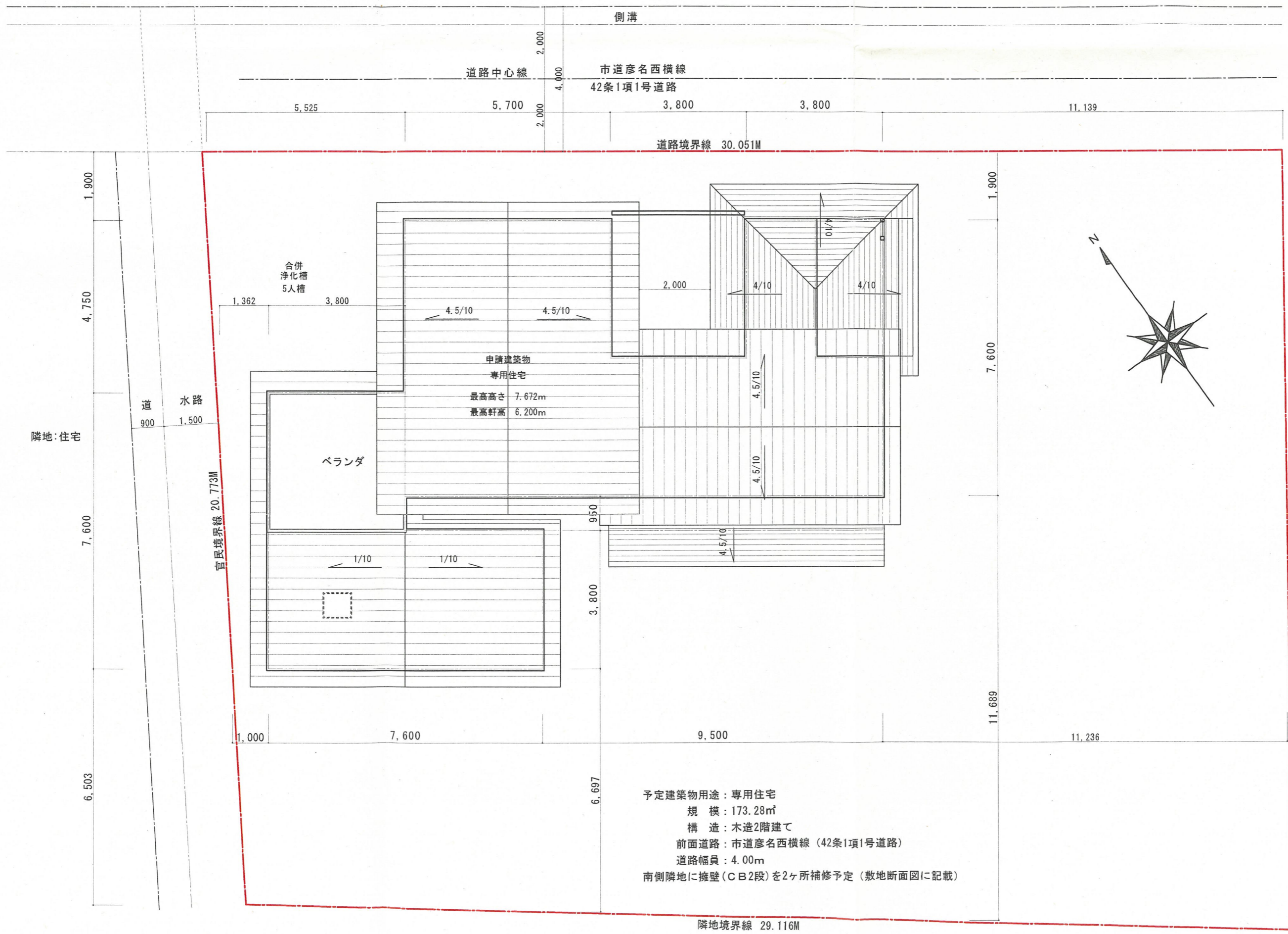
配置図兼屋根伏図 S=1:100
